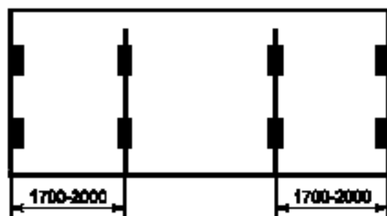
Рисунок В.2 — Размещение четырёх пар опорных площадок (одна пара на каждом торце плюс две промежуточные пары)
